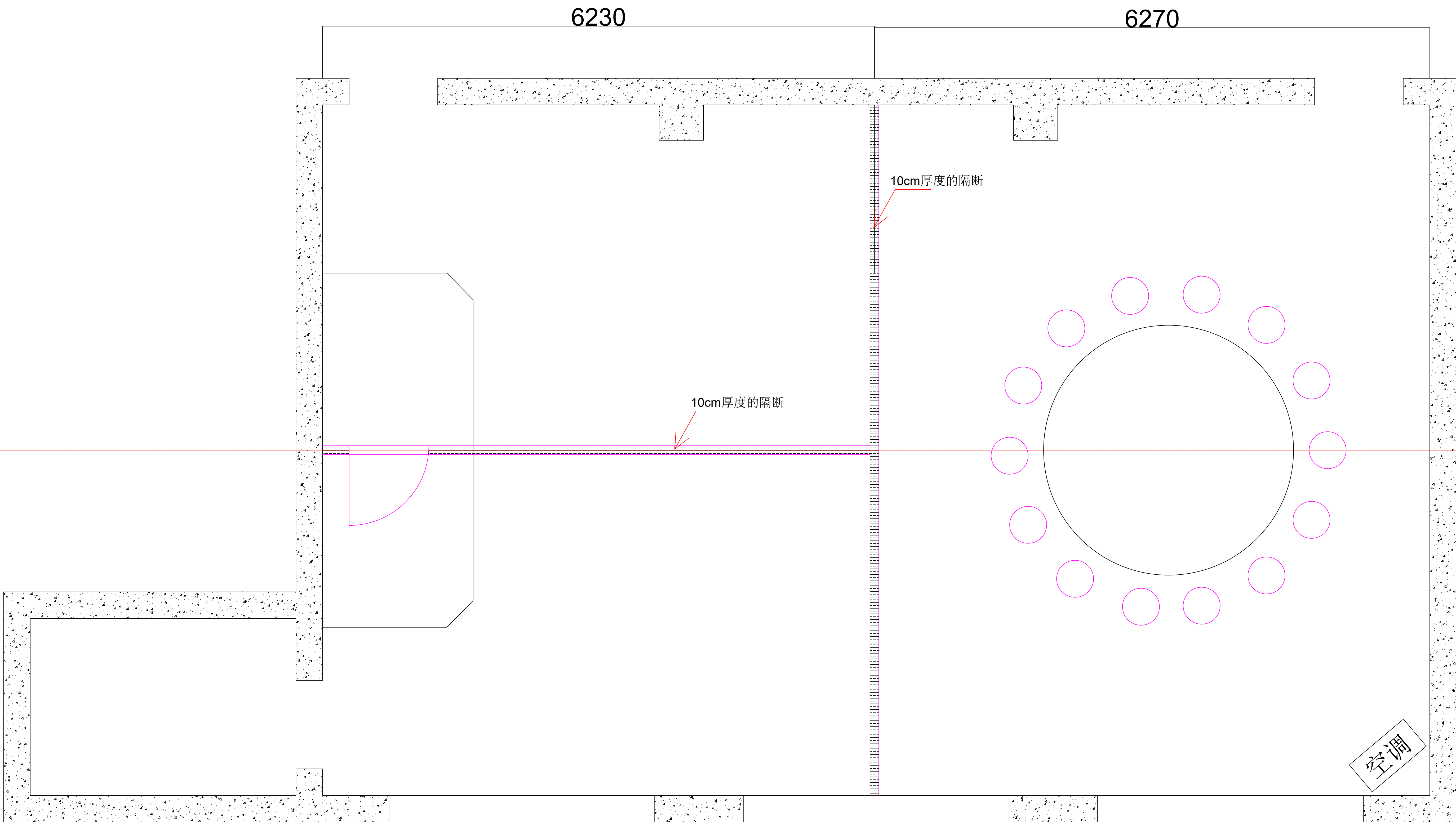
设计实训室弱电系统布线（含隔断）和家具的平面布置图
